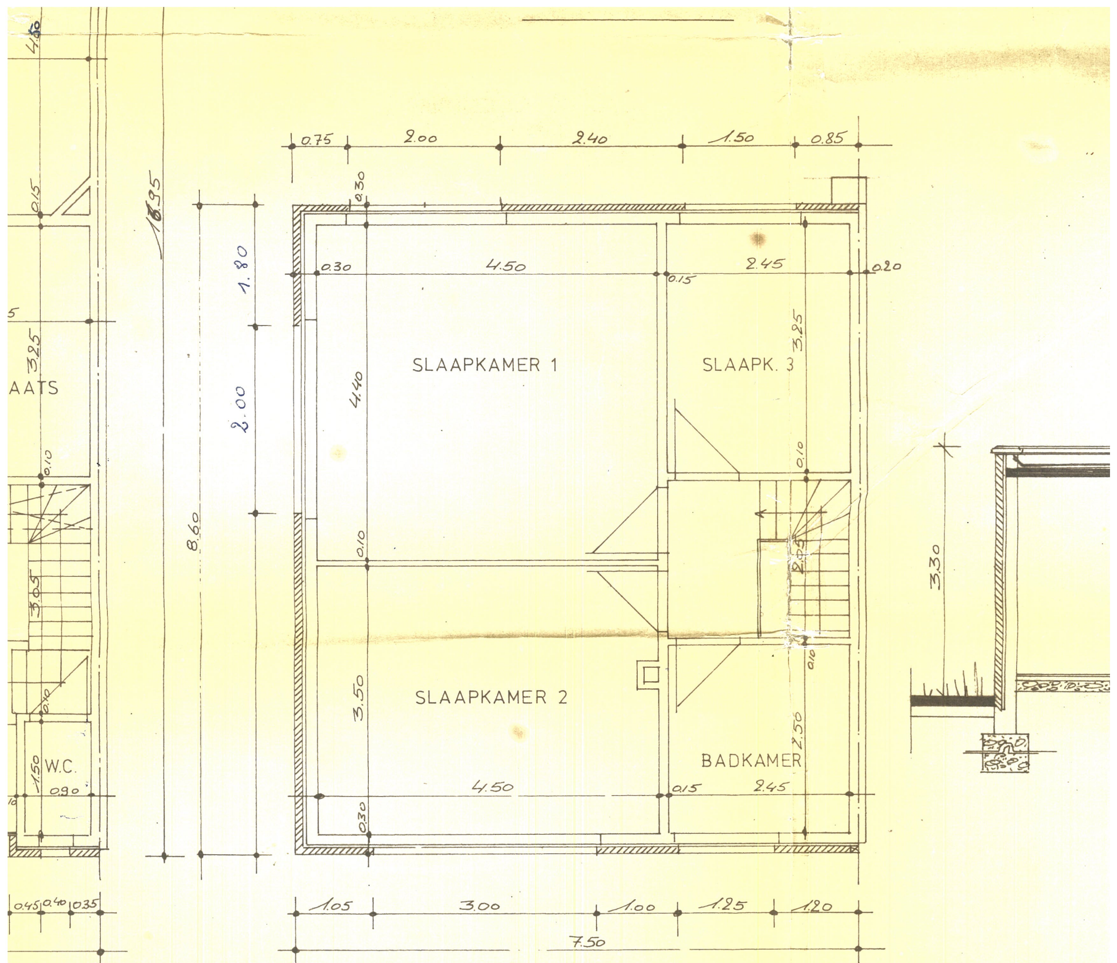
VERDIEPING
